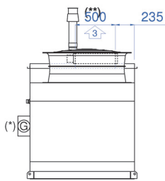
Vue de côté soufflage :
