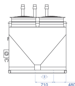
Vue de côté soufflage :
