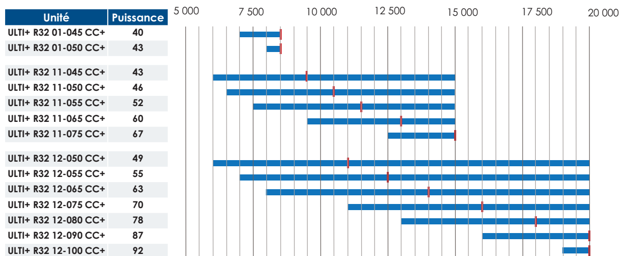
Plage de débit (m³/h) & débit nominal (l)
