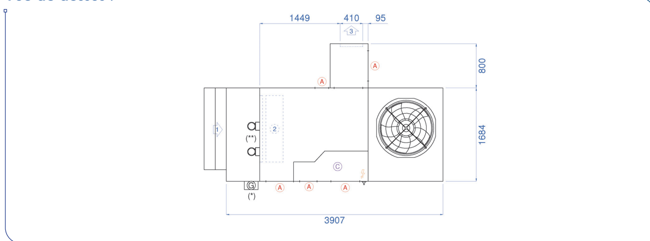
Vue de côté reprise :
