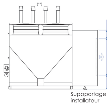
Vue de côté soufflage :
