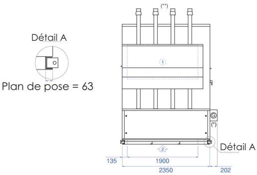
Vue de côté reprise :
