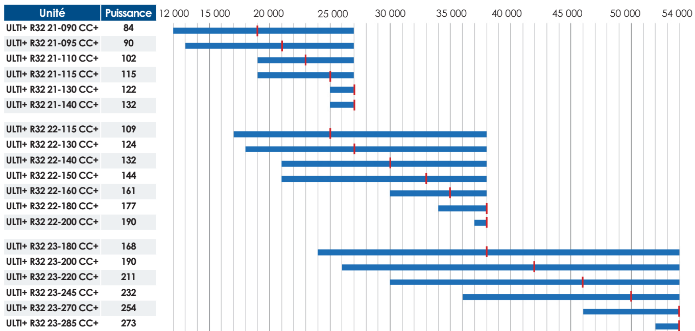
Plage de débit (m³/h) & débit nominal (l)
