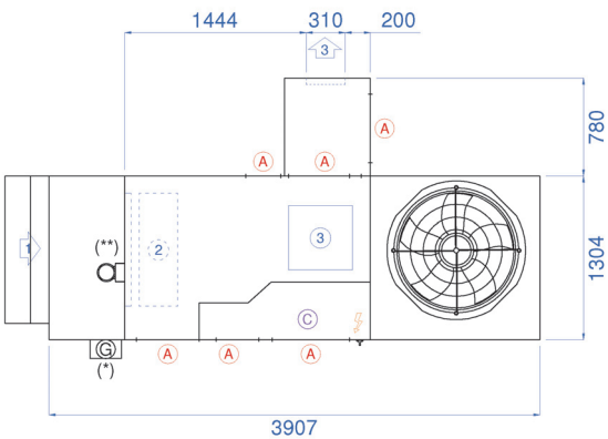
Vue de côté soufflage :
