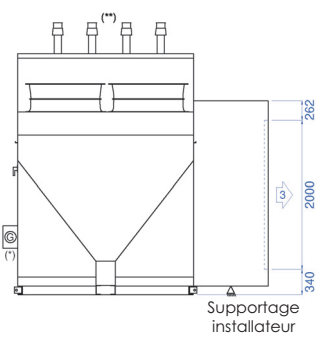
Vue de côté soufflage :
