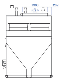
Vue de côté soufflage :
