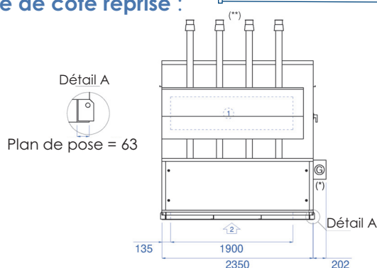
Vue de côté reprise :
