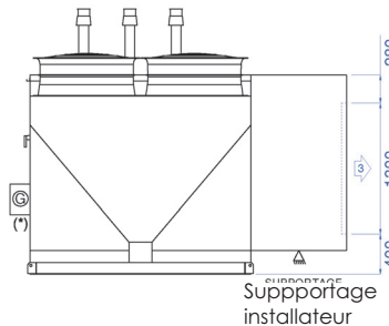
Vue de côté soufflage :
