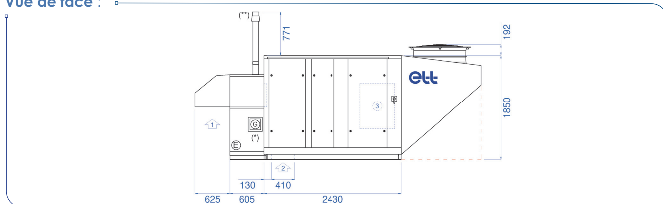
Vue de face :
