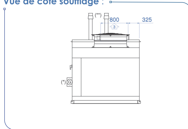
Vue de côté soufflage :
