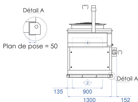
Vue de côté reprise :
