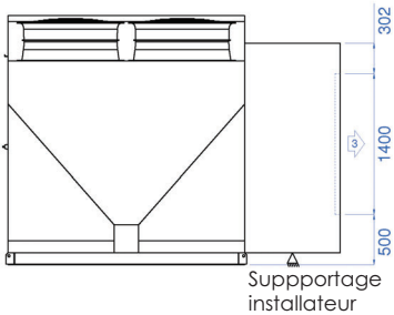
Vue de côté soufflage :
