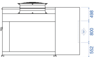
Vue de côté soufflage :
